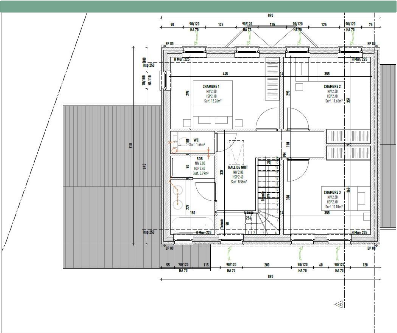
Plan Rez+1 Echelle 1/50
